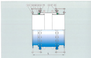
鋼製可撓管 (第2型)
